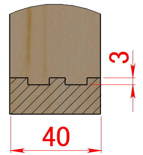
詳細図 B
