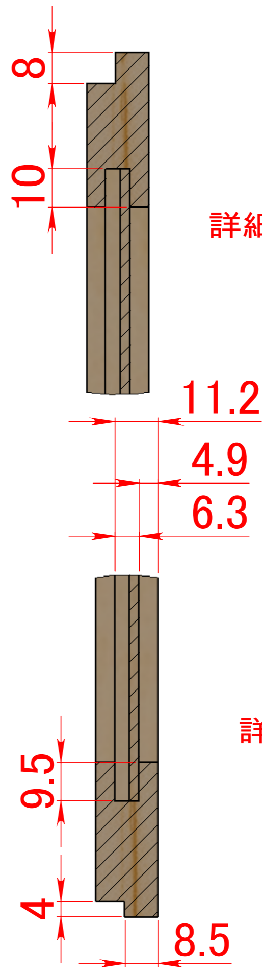
断面図 A-A
